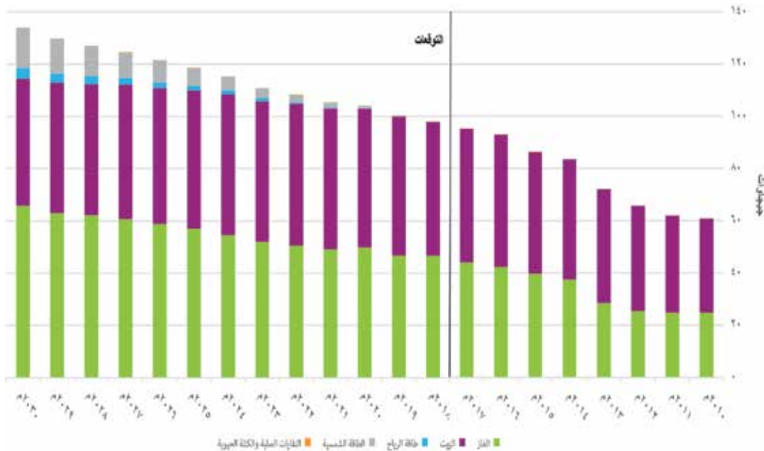
الشكل ١٢: الزيادة الفعلية والمتوقعة في الطاقة الاستيعابية لتوليد الكهرباء حسب نوع الوقود (بما في ذلك الغاز الطبيعي) المستخدم في المملكة خلال الفترة من عام ٢٠١٠م إلى عام ٢٠٣٠م
