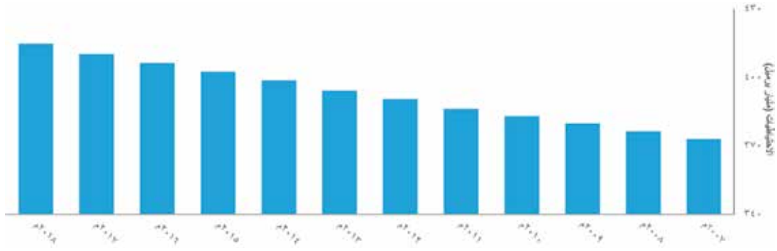
الشكل ١٤: احتياطات المملكة الأصلية من النفط الخام والمكثفات من عام ٢٠٠٧م حتى عام ٢٠١٨م
